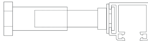
Führungsschiene mit Abstandhalter - Aufputz
