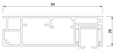
Exklusiv-Führungsschiene - Unterputz
